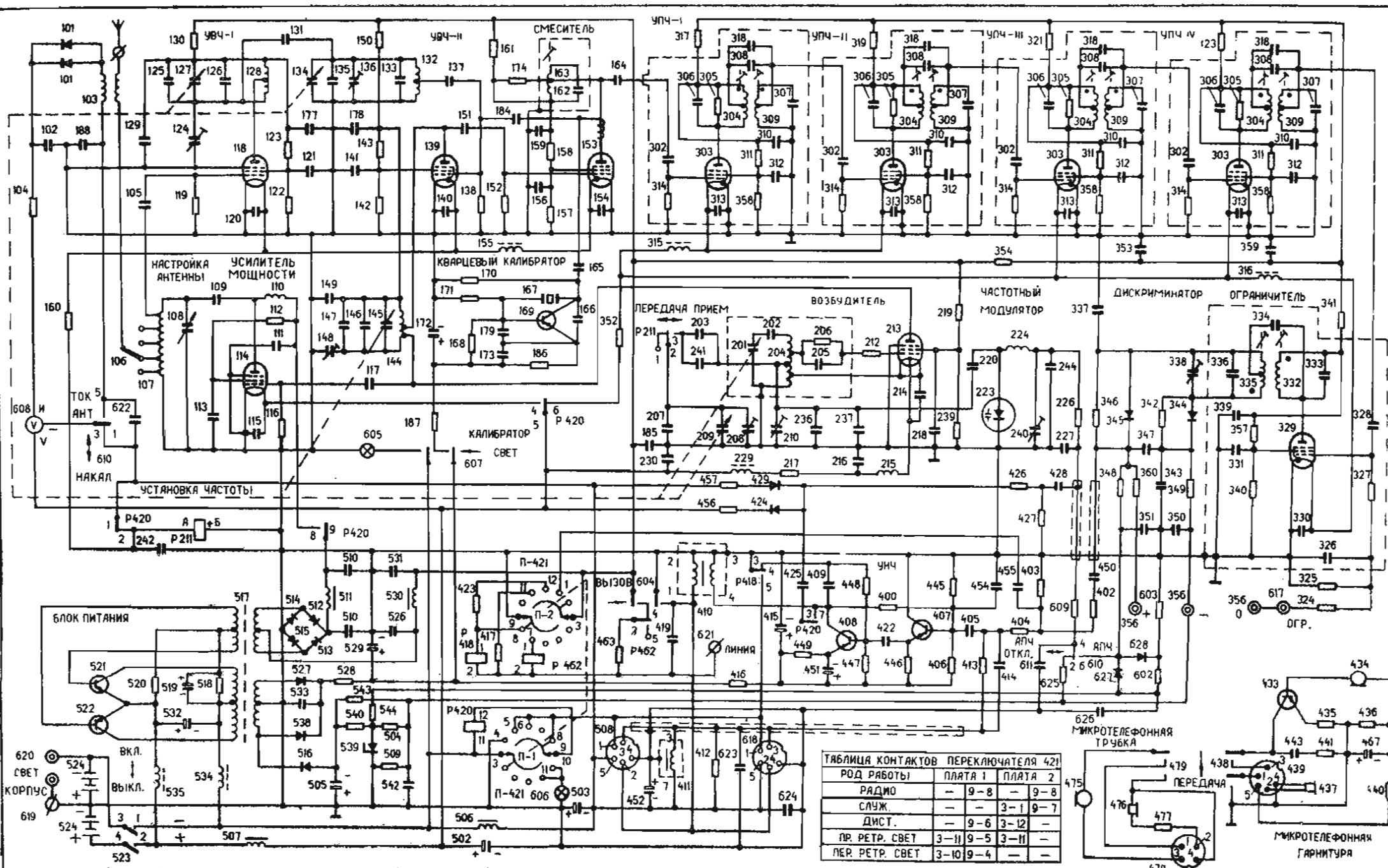
ПРИНЦИПАЛЬНАЯ СХЕМА РАДИОСТАНЦИИ
